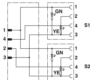
Схема расположения контактов вилки M12 и розетки M12, со светодиодами, с переключателем
