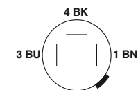
Расположение контактов разъема QUICKON, 3-полюсн.
