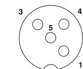
Расположение контактов гнезда M12, 4-контактное
