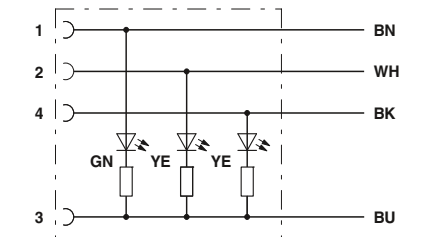
Цолевка контактов розетки M12 со светодиодным индикатором
