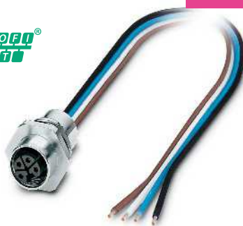
Кодировка L, сечение проводника: 2,5 мм 2 , 4-конт.
