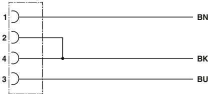
Цоколевка контактов розетки M12 с перемычкой
