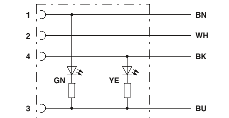
Цолевка контактов розетки M8/M12, со светодиодным индикатором
